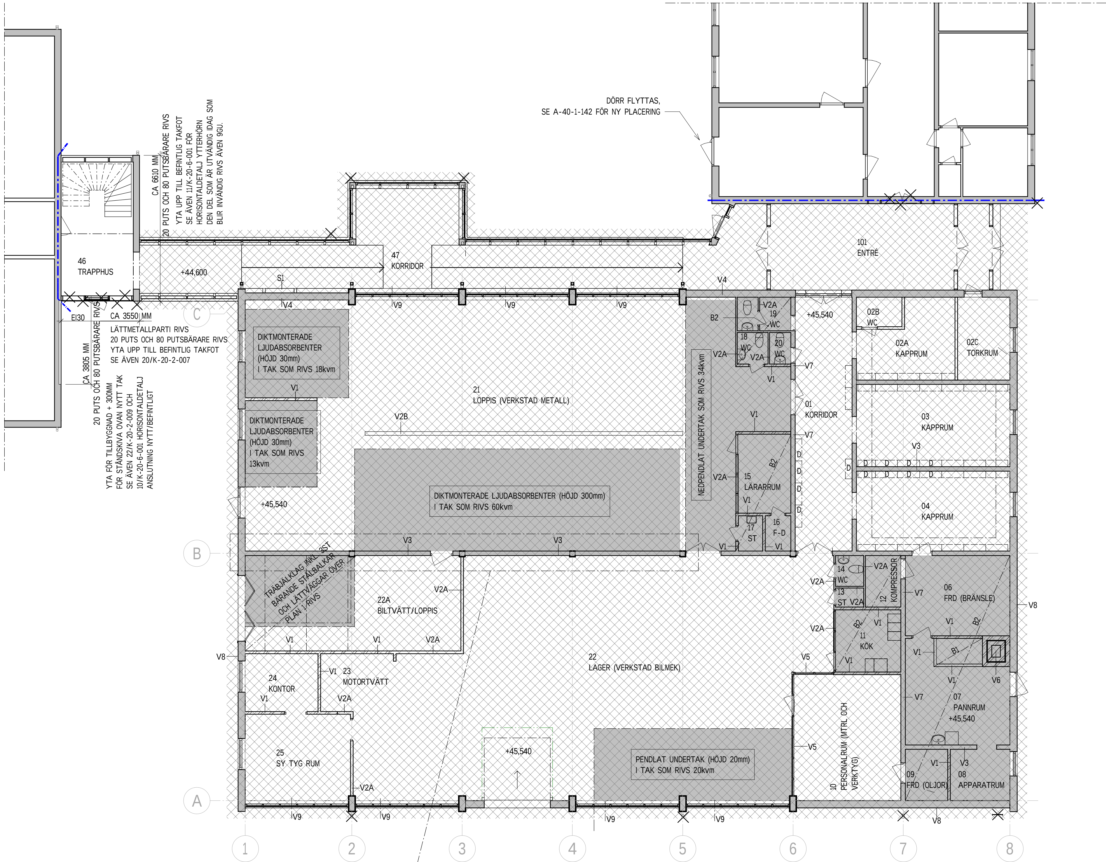
PLAN - BEFINTLIGA FÖRHÅLLANDEN, RIVNING 1 : 100
